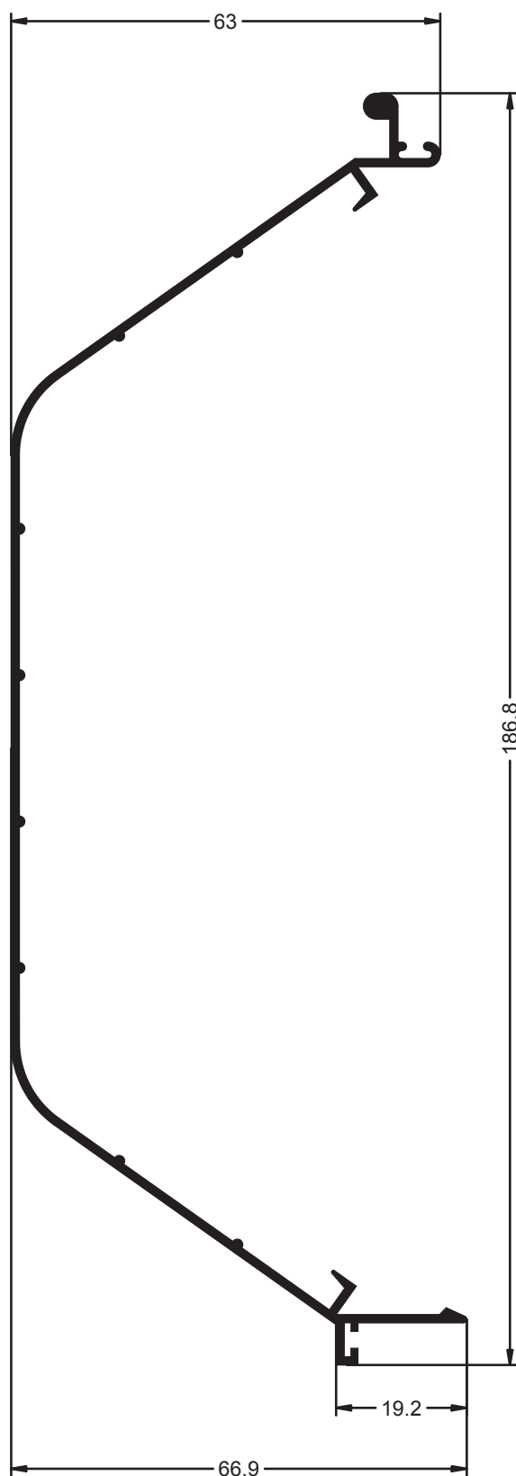
Ref.- 2569 Tapa Cajon Persiana con Aislante
