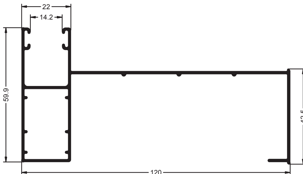
Ref.- 2570 Mainel Monoblock
