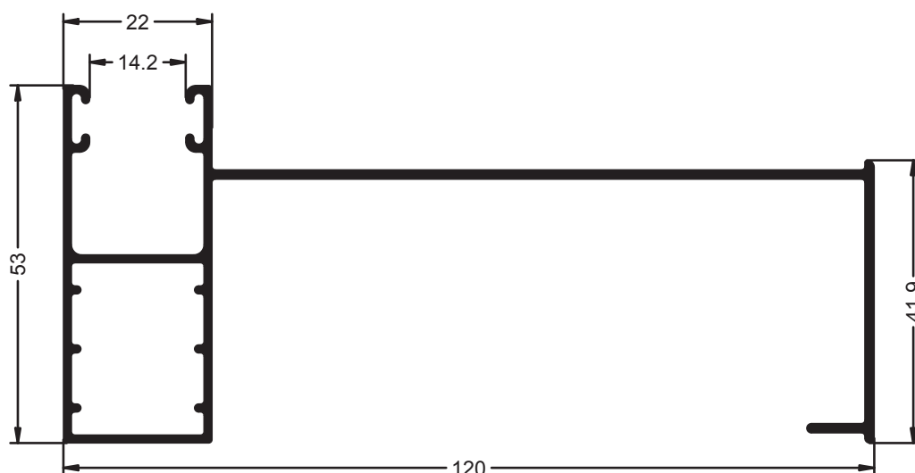
Ref.- 2547 Mainel Monoblock
