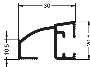
Ref.- 2590 Tapajunta de Mainel
