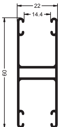
Ref.- 1539 Guia Persiana Doble
