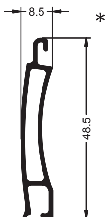
Ref.- 2422 Lama de Persiana Mini
