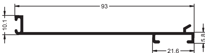
Ref.- 2576 Cortavientos Persiana
