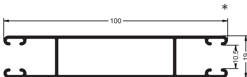
Ref.- 2431 Guia Persiana Doble
