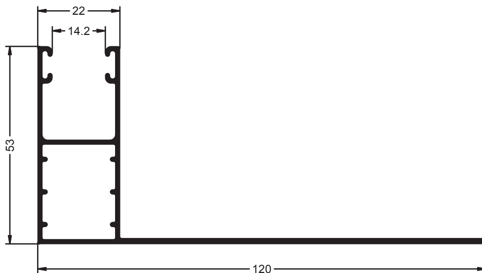
Ref.- 2537 Mainel Monoblock
