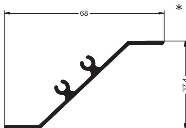
Ref.- 2520 Lama para Celosia
