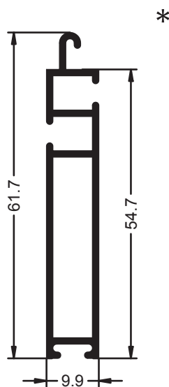
Ref.- 2449 Terminal de Persiana
