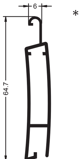
Ref.- 7143 Lama de Persiana
