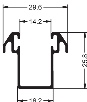
Ref.- 2508 Guía de Persiana
